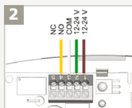
De draden als volgt verbinden: 1 - BRUIN - VOEDING 2 - GROEN - VOEDING 3 - WIT - COM 4 - GEEL - NO 5 - GEEL - NC
