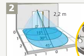
Pas de verticale hellingshoek van de antenne aan.
