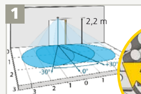
Pas de zijdelingse hellingshoek van de antenne aan.
